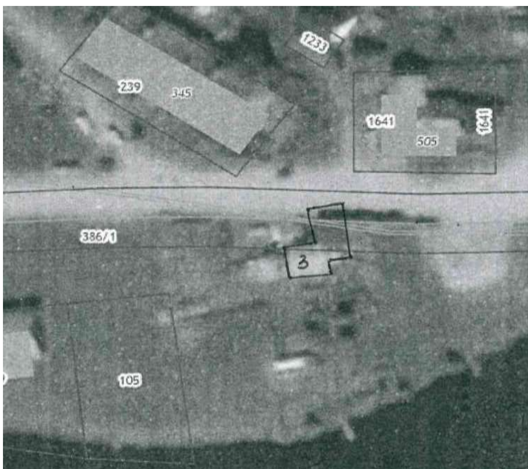
схема расположения
